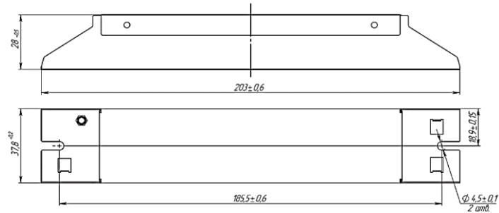
а) Блок аварийного питания
