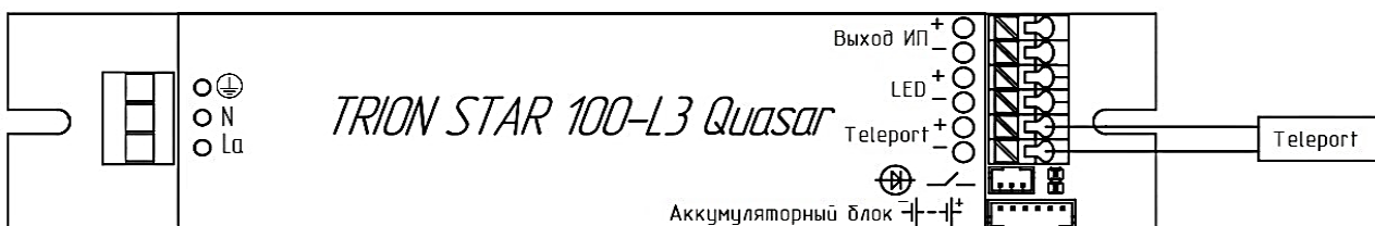
Рисунок 5 – Схема подключения УДТУ «Teleport»
