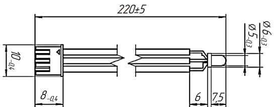
в) LED-индикатор
