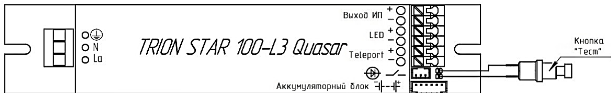
Рисунок 4 – Схема подключения кнопки «Тест»
