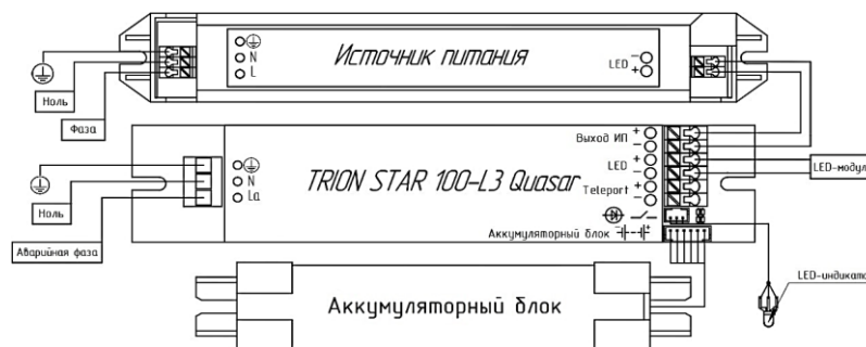
Рисунок 3 – Схема подключения БАП
