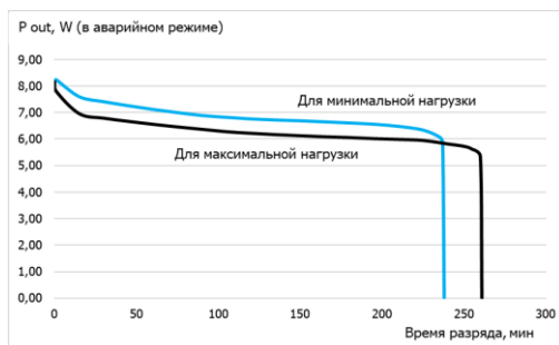
Рисунок 2 – Зависимость мощности в аварийном режиме от времени разряда (на max и min нагрузке)
